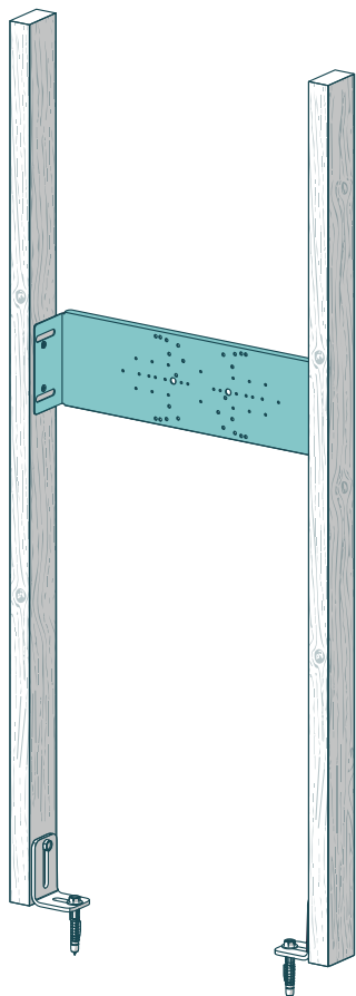
Монтаж в деревянный каркас
